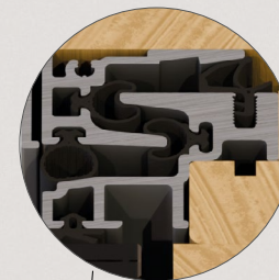
NODO CENTRALE 38MM CON SISTEMA LABIRINTO PER FAVORIRE LA CHIUSURA.
