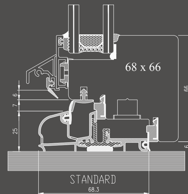
Nodo inferiore portafinestra con soglia
