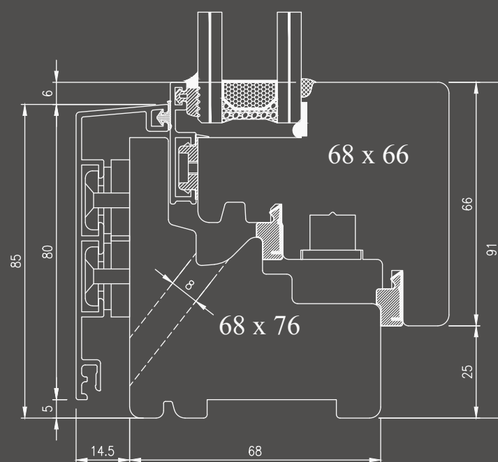
Nodo inferiore finestra
