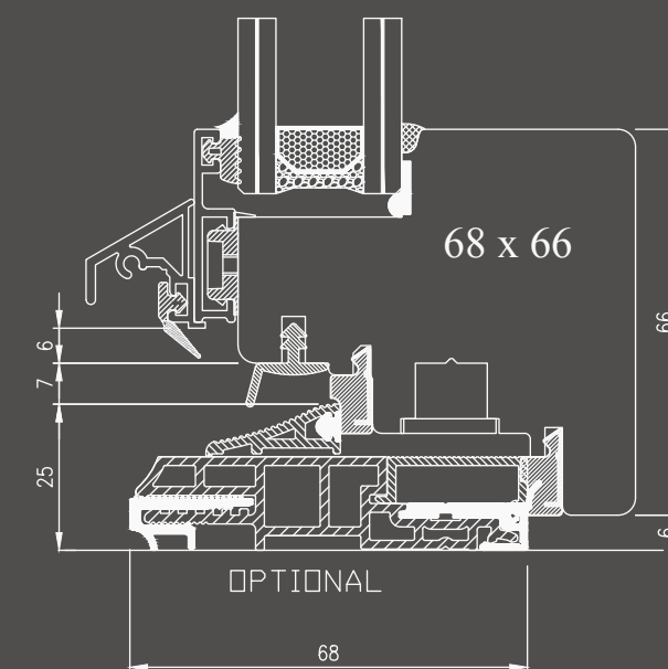
Nodo inferiore portafinestra con soglia
