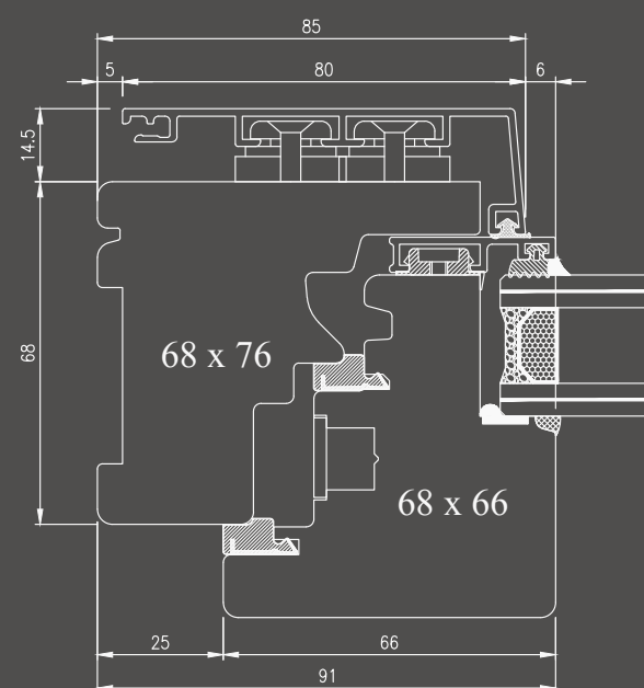
Nodo superiore/laterale finestra e portafinestra
