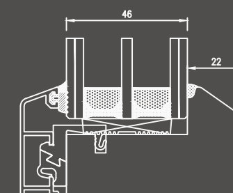
SMUSSATO
