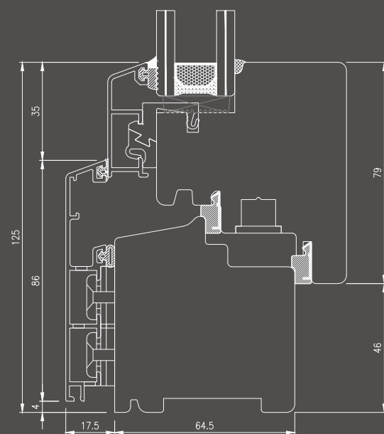
Nodo inferiore standard finestra Gocciolatoio solidare
