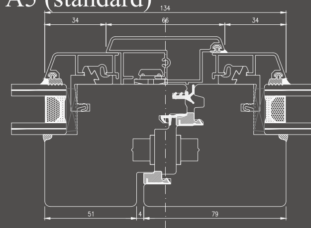
A5 (standard)
