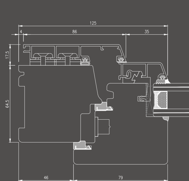
Nodo superiore/laterale finestra e portafinestra
