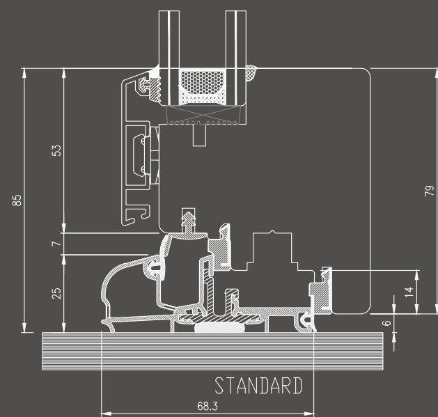
Nodo inferiore portafinestra con soglia
