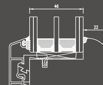
ARROTONDATO
