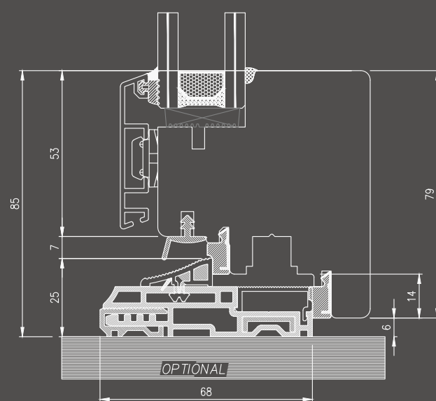
Nodo inferiore portafinestra con soglia
