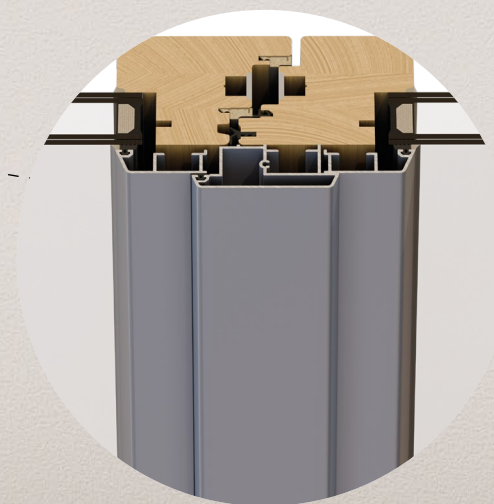
NODO CENTRALE LATO ESTERNO. DISPONIBILI IN 3 VERSIONI.
