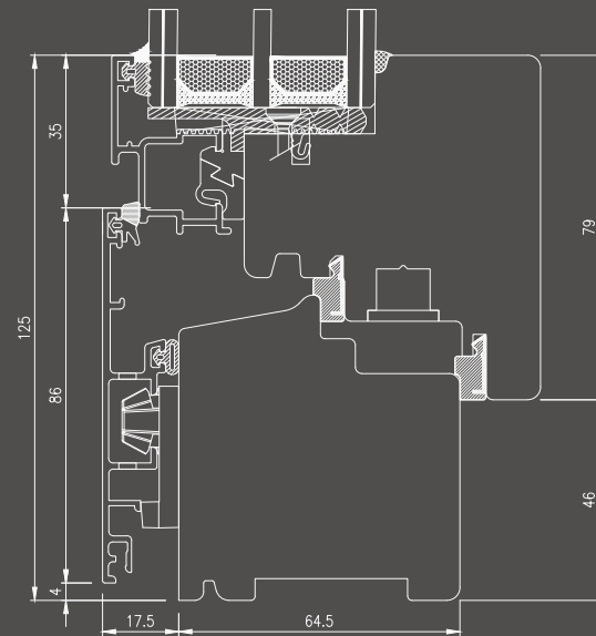
Nodo inferiore standard finestra Gocciolatoio solidare
