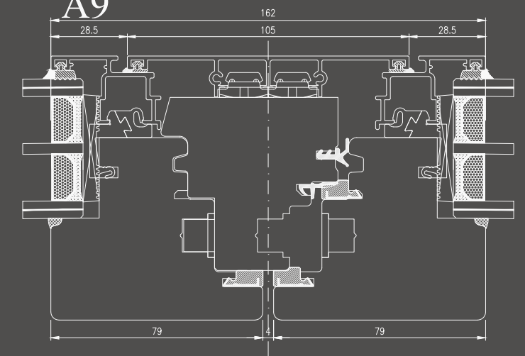
Nodi centrale di finestra/portafinestra
