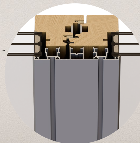
NODO CENTRALE COMPLANARE LATO ESTERNO
