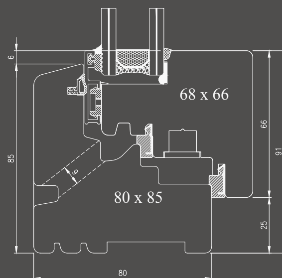
Nodo inferiore finestra
