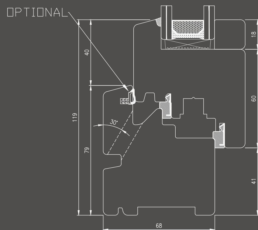
Nodo inferiore standard finestra gocciolatoio solidare
