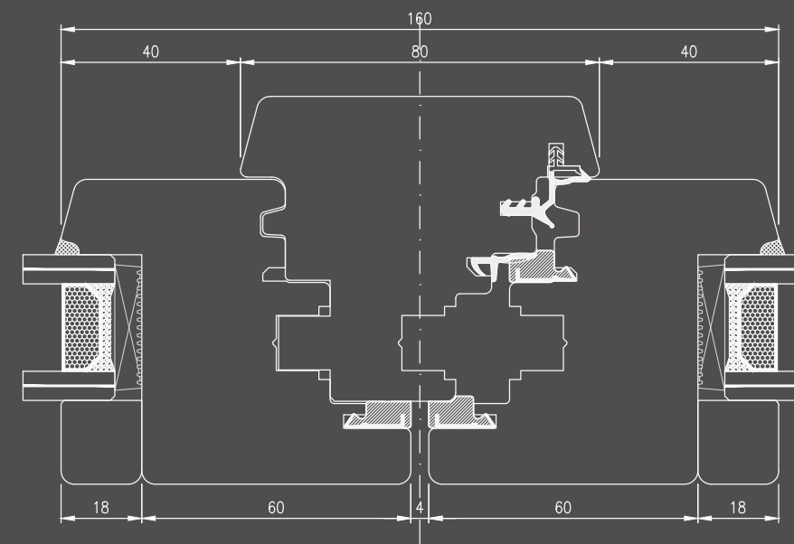
A9 Nodo centrale di finestra e portafinestra
