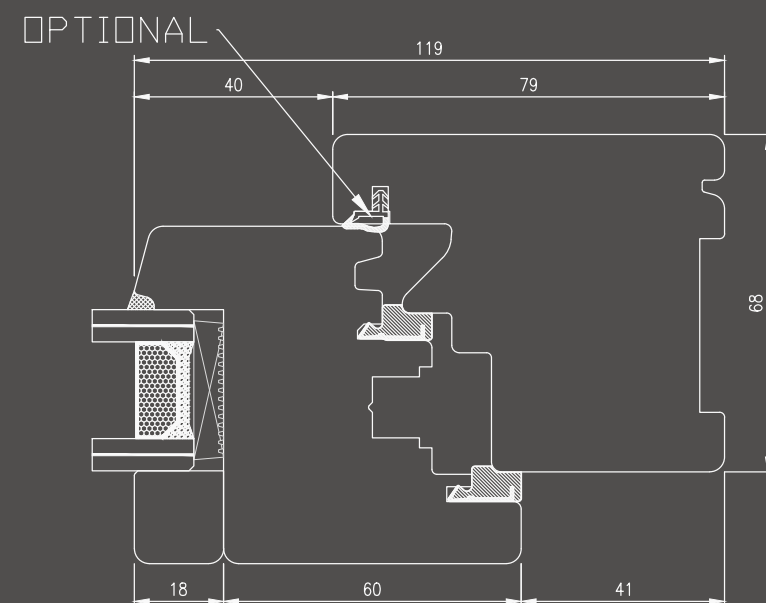
Nodo superiore/laterale finestra e portafinestra
