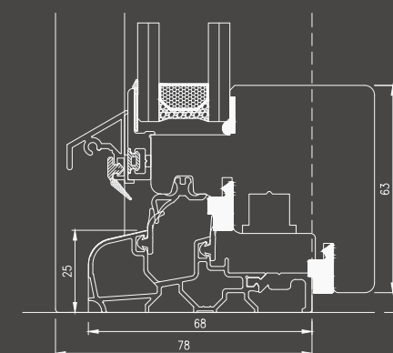
Nodo inferiore portafinestra con soglia
