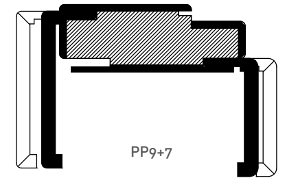
STIPITE DI SERIE (ad esclusione delle finiture Ciliegio I61, Noce tanganica I60 e Noce nazionale I59 con telaio PP7+7)
