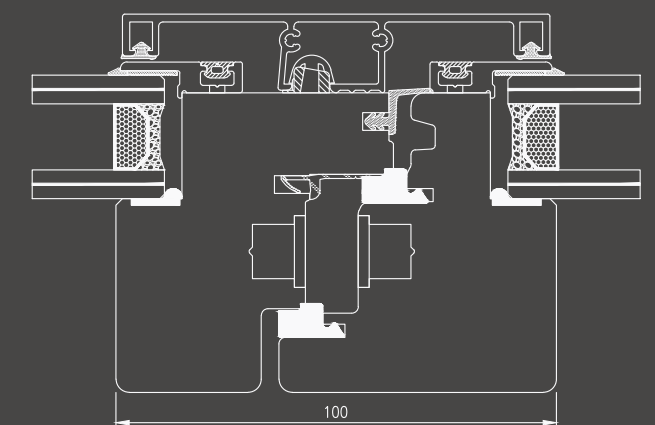
Nodo centrale di finestra/porta
