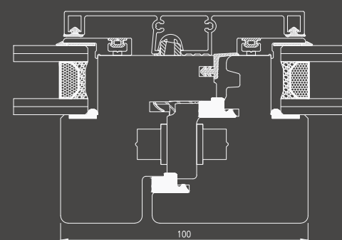
Nodo centrale con profilo in alluminio (standard) di Finestra/portafinestra
