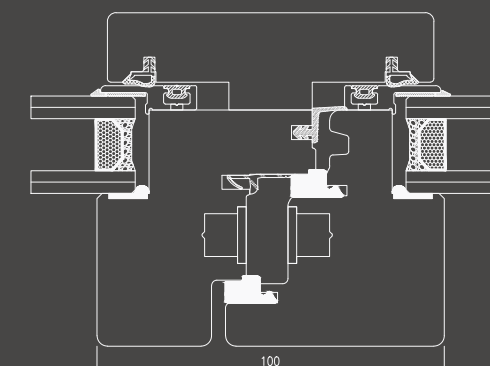
Nodo centrale con profilo esterno in legno (optional) di finestra/portafinestra
