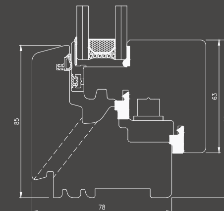
Nodo inferiore finestra
