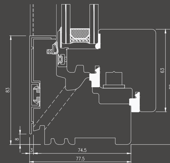
Nodo inferiore finestra
