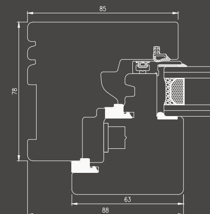
Nodo superiore/laterale finestra e portafinestra
