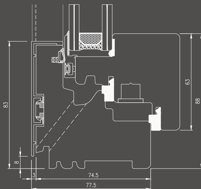
Galce inferior ventana
