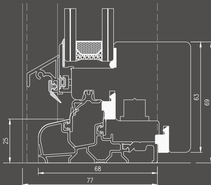
Galce inferior balconera con solera
